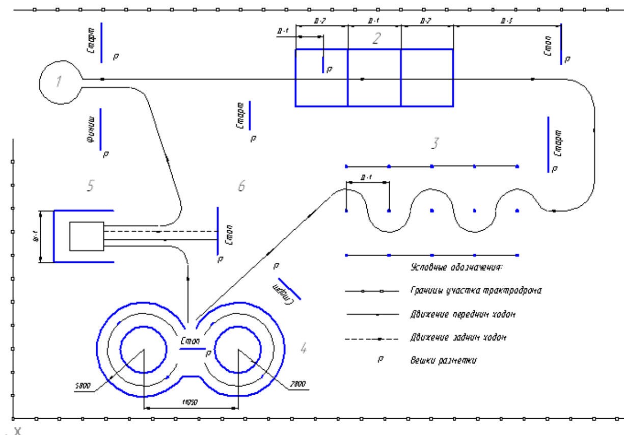
Рисунок 1- Схема маршрута движения на трактородроме
